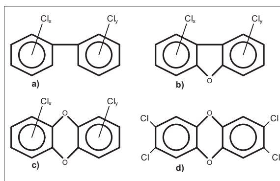
Ryc. 1. Wzory strukturalne przedstawicieli poszczególnych grup TZO; a) – polichlorobifenyli (PCB), b) – polichlorodibenzofurany (PCDF), c) – polichlorodibenzodioksyny (PCDD), d) – 2,3,7,8-tetrachlorodibenzo- p -dioksyna (TCDD)
