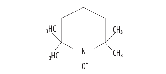
Ryc. 1. Stabilizacja rodnika nitroksydowego (Tempo), pochodnej 2,2,6,6-tetrametylopiperydyny przez grupy metylowe
