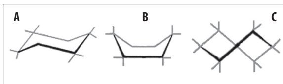
Ryc. 4. Konformacje nitroksydów piperydynowych: A – krzesetkowa, B – łódkowa, C – skręcona
