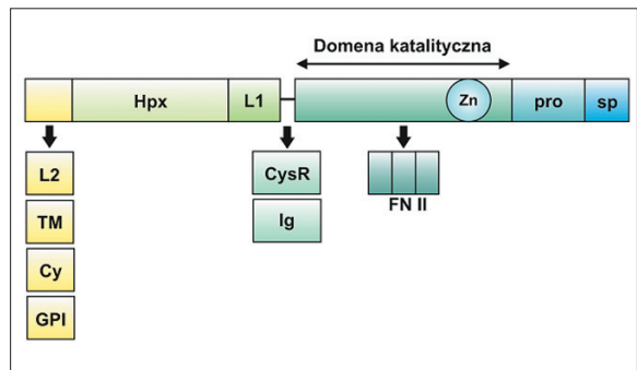
Ryc. 2. Budowa domenowa metaloproteinaz macierzowych; L1, L2 – fragmenty łącznikowe; TM – domena transmembranowa; Cy – ogon cytoplazmatyczny; GPI – glikozylfosfatydyloinozylol; Hpx – domena hemopeksynowa; CysR – domena bogata w reszty cysteiny; Ig – domena immunoglobulinowa; FNII – trzykrotnie powtórzony motyw fibronektyny typu II; Zn – atom cynku; pro – propeptyd; sp – peptyd sygnałowy
