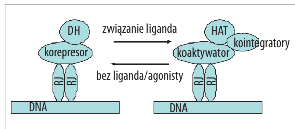
Ryc. 1. Schemat reorganizacji struktury kompleksu czynników transkrypcyjnych aktywowanych ligandem; RJ – receptor jądrowy, DH – deacetylaza histonów, HAT – acetylotransferaza histonów
