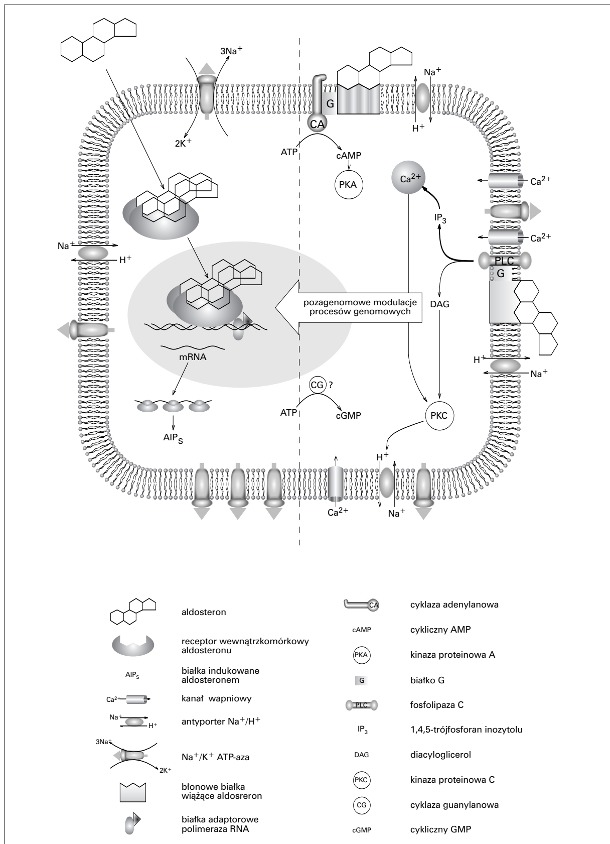
Ryc. 2. Dwustopniowy model działania aldosteronu. Schemat przedstawia pozagenomowe (szybkie) mechanizmy działania aldosteronu (strona prawa) oraz genomowe (opóźnione) oddziaływania poprzez receptory wewnątrzkomórkowe (strona lewa)
